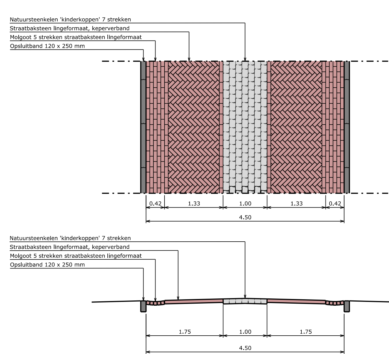
Doorsnede Spijkert / Hoog mikkert Schaal 1:50
