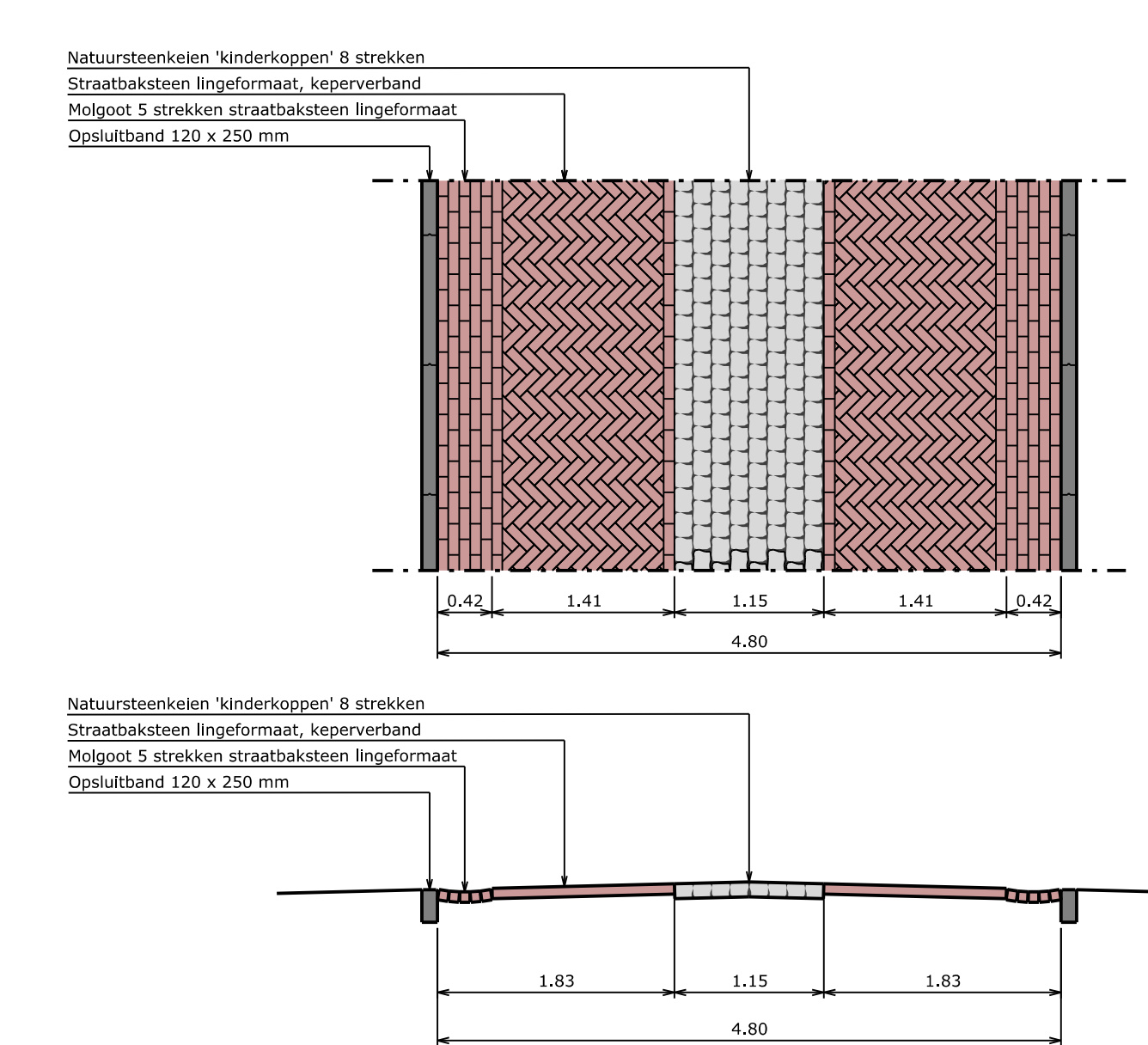
Doorsnede Eeneind / Eeuwdrissenstraat / Oudedijk Schaal 1:50
