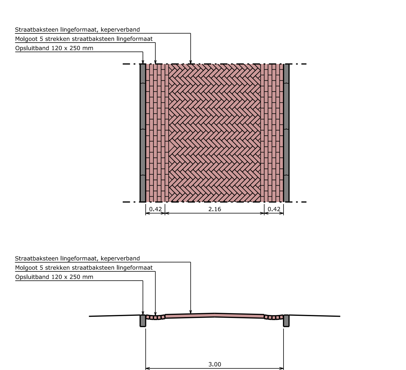
Doorsnede Molekeslaan Schaal 1:50
